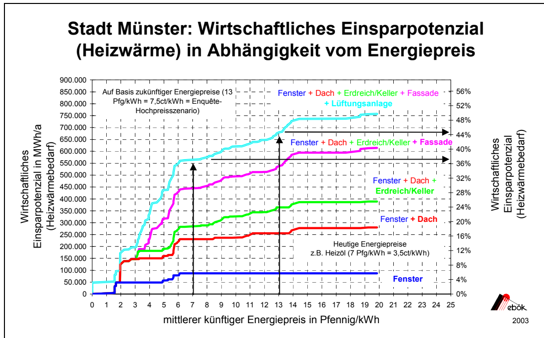
Abb. 8: Einsparpotentiale verschiedener Wärmedämm-Maßnahmen in Abhängigkeit von den spezifischen Energiekosten
