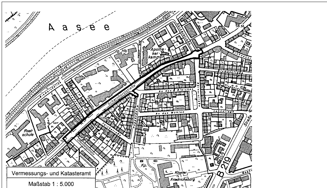
Übersichtsplan Nr. 1 zur Offenlegung des Ausbauplanes für die Anlegung von Parkstreifen in der Scharnhorststraße
