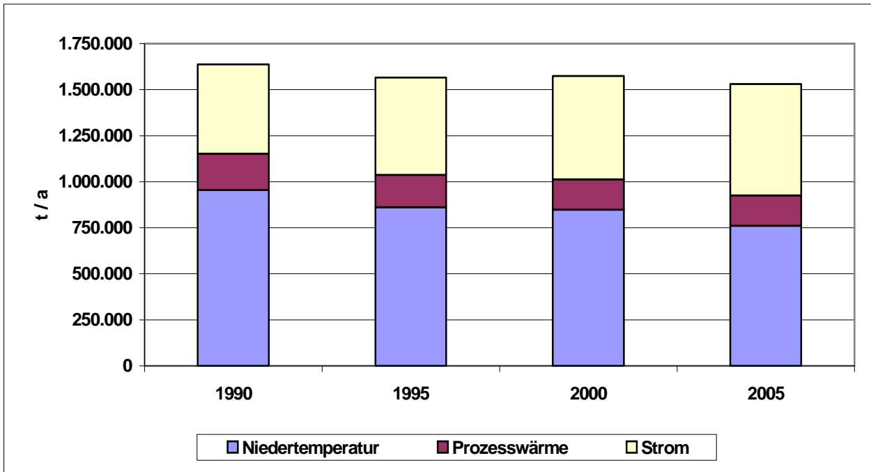
Abbildung 2: CO 2 -Emissionen im Energiesektor, 1990 bis 2005
